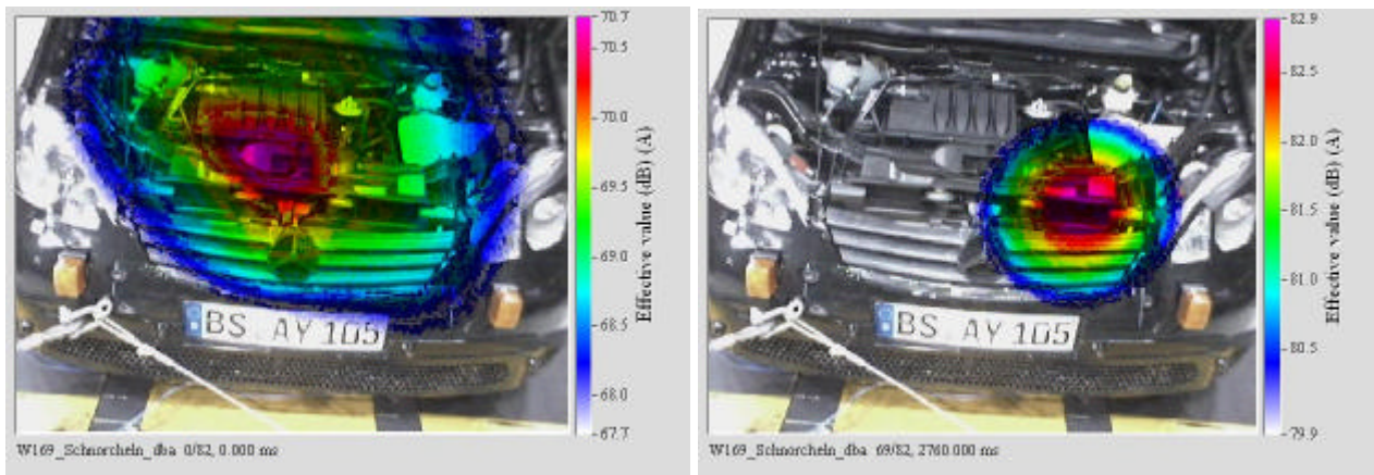
Bild 7: Schallbilder: links Leerlaufgeräusch, rechts Schnorcheln beim Abtounen
